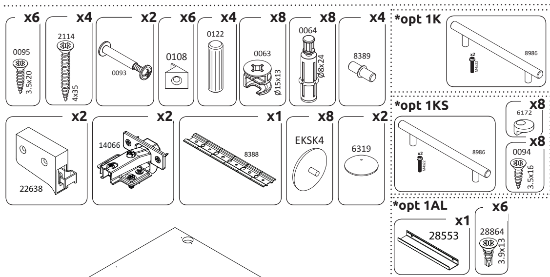
V5-60-1KS 600x540x320
